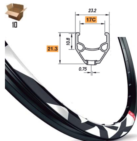
R0465C0011P90M2215593203.....21,60 € LLANTA 26" MACH1 MX DISC (559 x 17C) ALUMINIO 32H. ERD 534 mm. Negra
