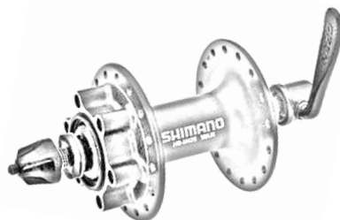
R3211C0009P60AHBM475BL.....17,50 € BUJE DELANTERO M475 32H. DISCO 6 TORNILLOS. Negro
