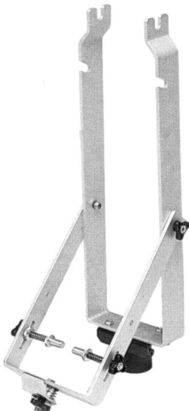
R0169C0051P4992480.....93,00 € CENTRADOR DE RUEDA AL BANCO
