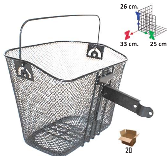
R2538 C0007P84A038H..... 14,20 € CESTA METÁLICA DELANTERA EXTRAIBLE CON ASA Y SOPORTE A LA CAÑA POTENCIA (Ø 22,2 mm.) 26 x 33 x 25 cm. Negra
