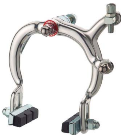
R0651C0003P48HJ1020A.....6,40 € PUENTE FRENO BALON ALUMINIO 73-91 mm. Delantero ó Trasero
