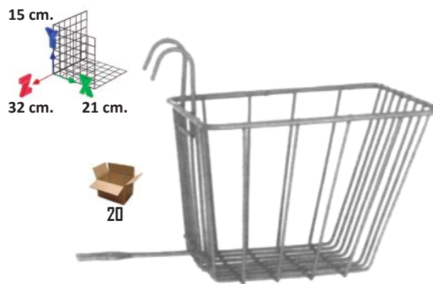
R0419C0005P3617.....9,80 € CESTA METÁLICA DELANTERA EXTRAIBLE MEDIANA CON CANCHOS AL MANILLAR 15 x 32 x 21 cm. Blanca
